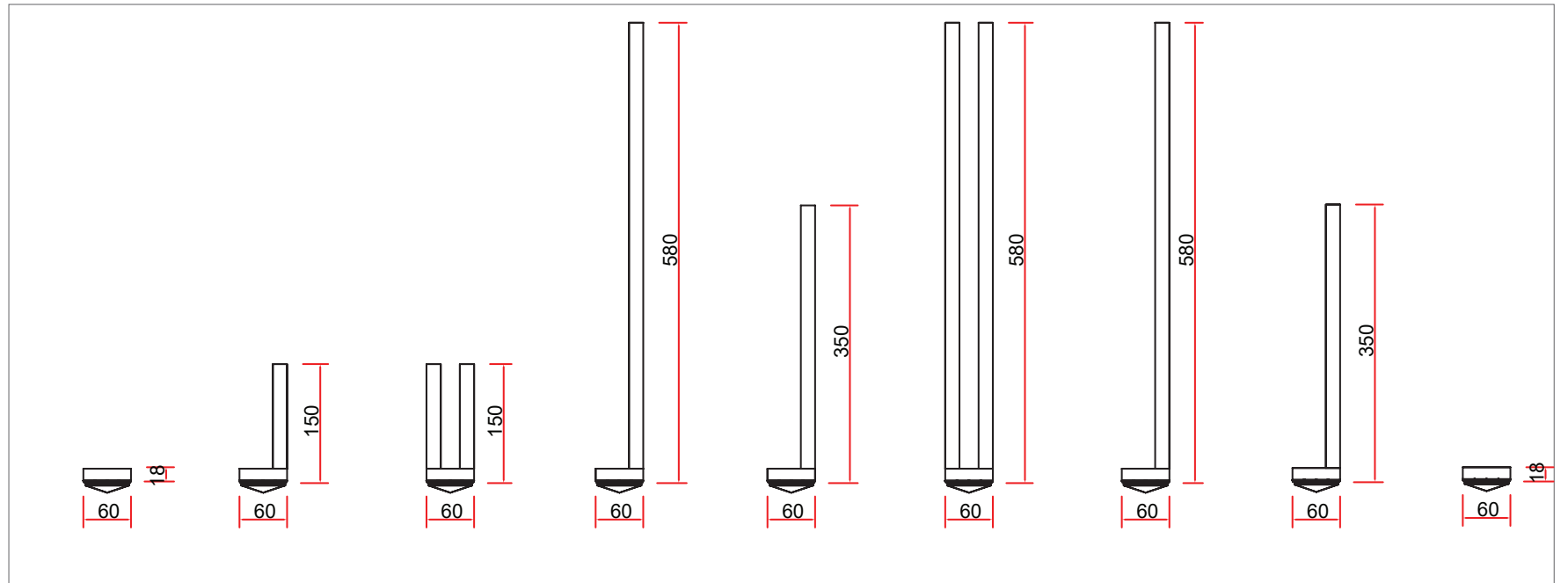
DEKOR PANELLER KESİT ÖLÇÜLERİ
